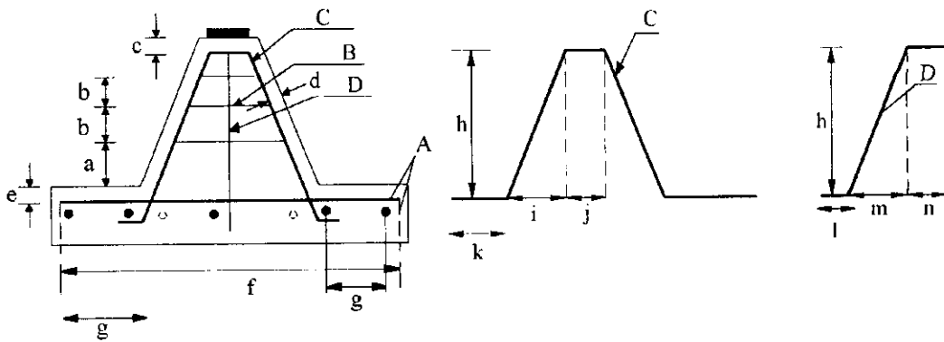
شکل ۱۳-۱۵- آرماتورهای فونداسیونها
