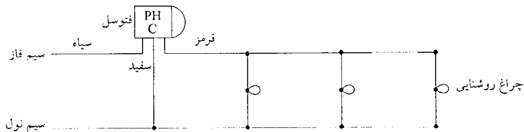
شکل ۱۴-۶- دیاگرام مدار فرمان تعدادی چراغ روشنایی به کمک عملکرد مستقیم فتوسل
